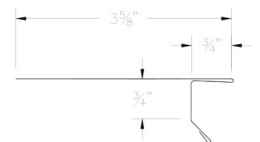
⑥① Drip Edge (ABSDcc)
